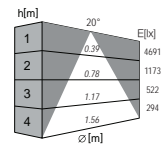
COB Module CRI95 20°
